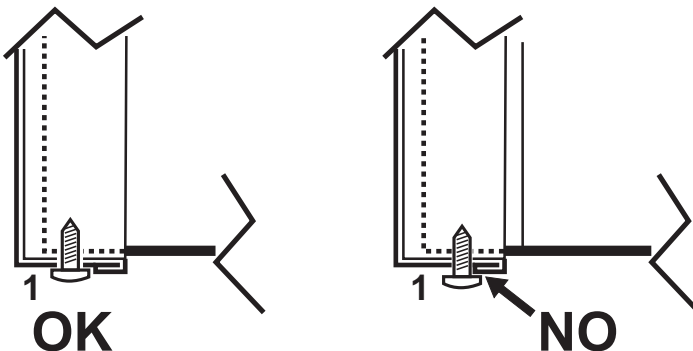
fig. 42 - Posizione corretta pannello frontale
