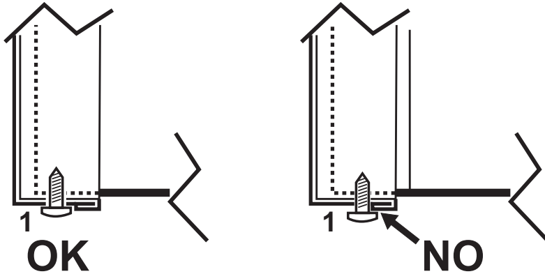
εικ. 42- Σωστή τοποθέτηση μπροστινού πίνακα
