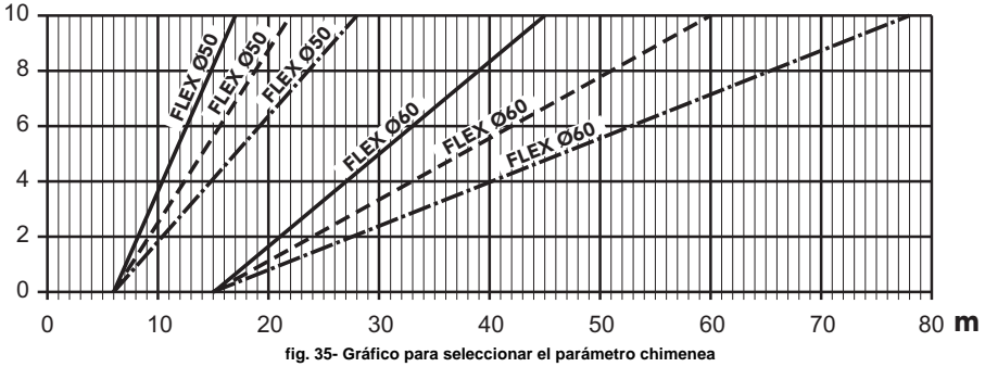
fig. 35- Gráfico para seleccionar el parámetro chimenea
