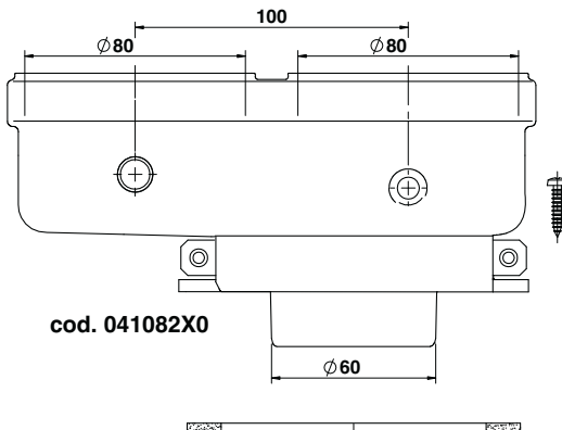
εικ. 33- Εξάρτημα σύνδεσης για ξεχωριστούς αγωγούς
