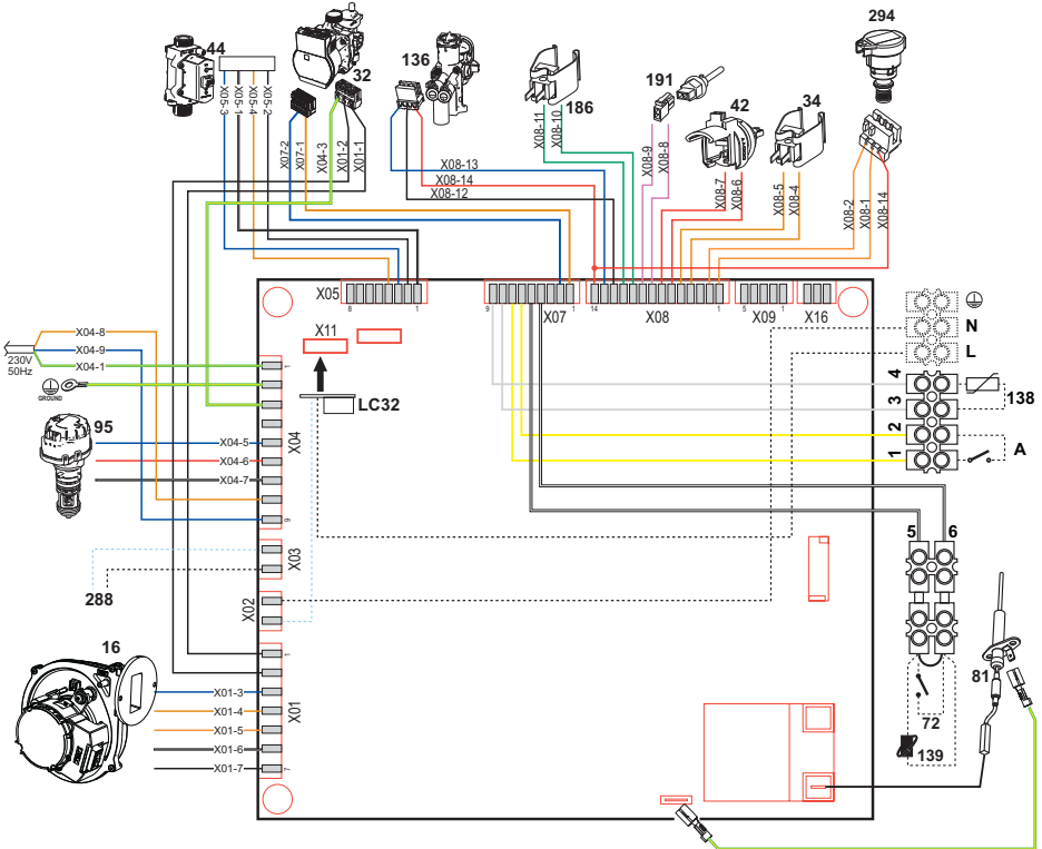
εικ. 67- Ηλεκτρολογικό διάγραμμα
