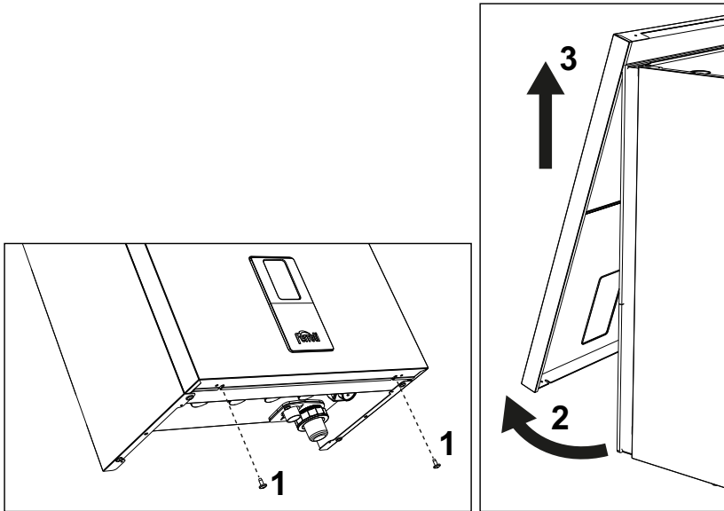
fig. 41 - Apertura pannello frontale
