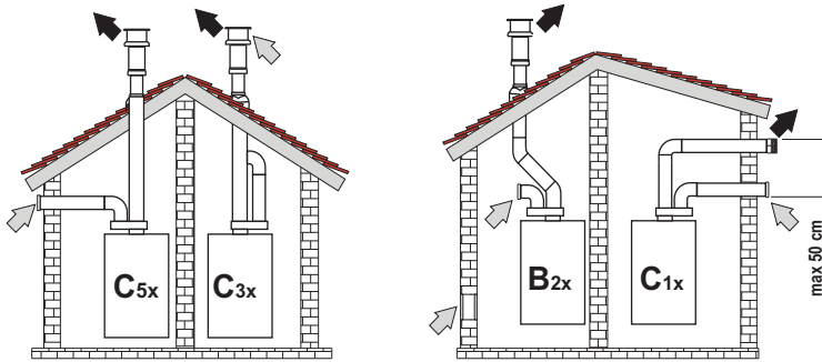
εικ. 32- Παραδείγματα σύνδεσης με ξεχωριστούς σωλήνες (⇨ = Αέρας / ⇩ = Καυσαέρια)
