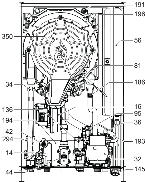
fig. 62 - Vista generale
