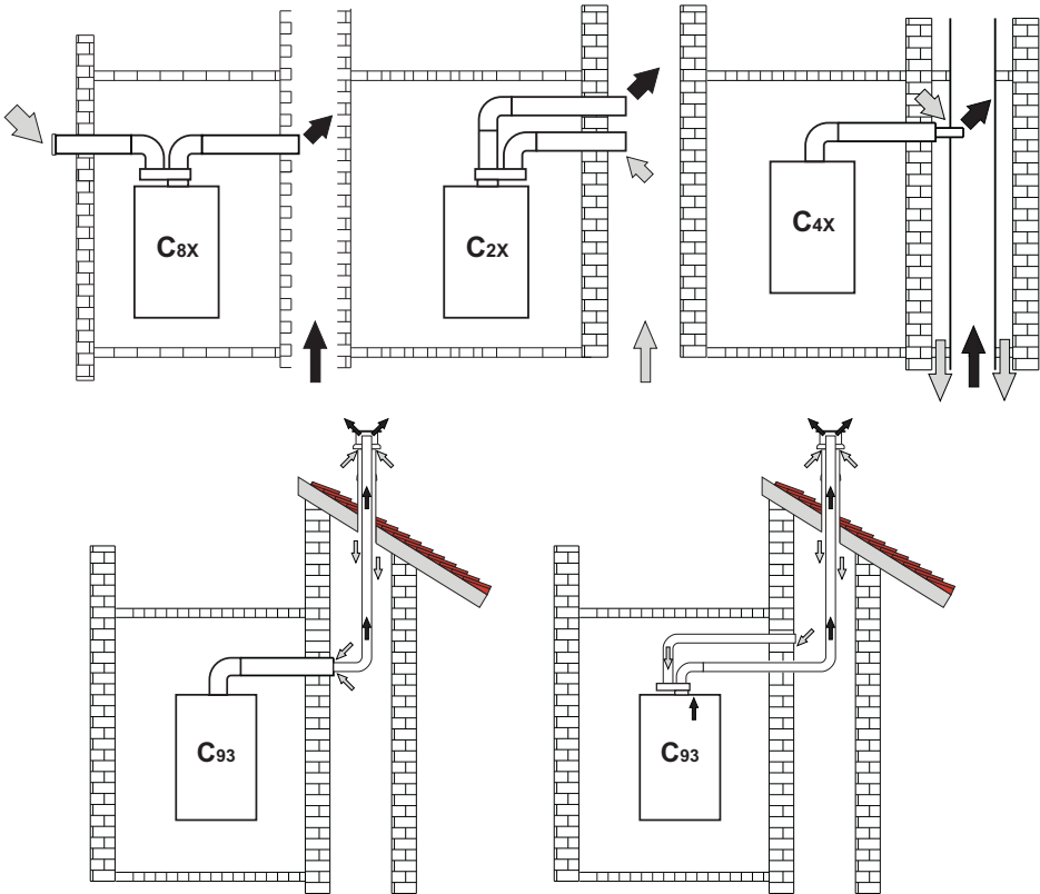
fig. 36 - Esempi di collegamento a canne fumarie (⇨ = Aria / ⇨ = Fumi)
